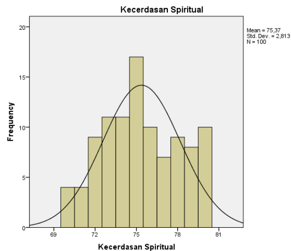
Gambar 2 Histogram Skor Hasil Tes Kecerdasan Spiritual
