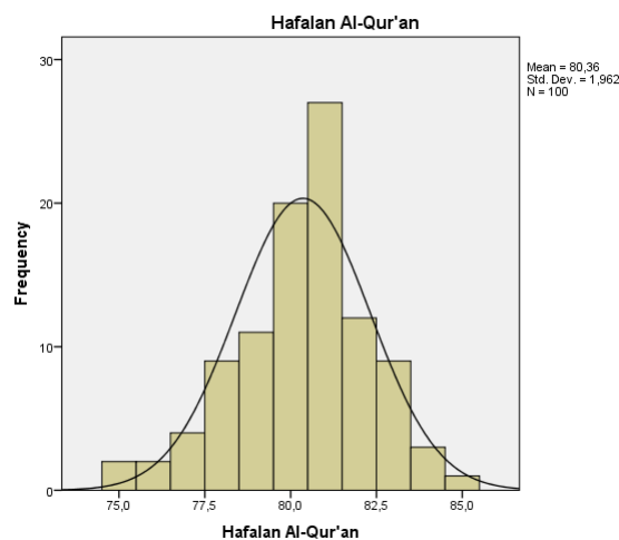
Gambar 1 Histogram Skor Hasil Tes Hafalan AL-Qur'an
