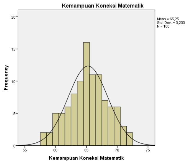
Gambar 3 Histogram Skor Kemampuan Koneksi Matematik
