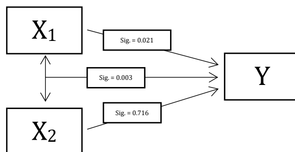
Gambar 4. Analisis Regresi Berganda
